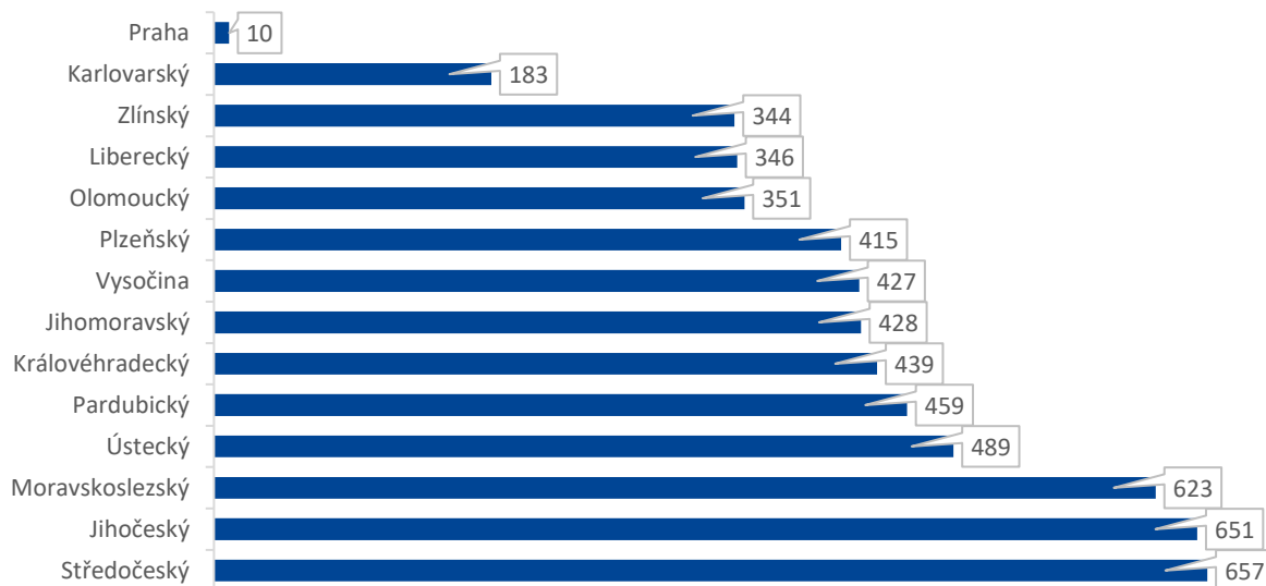
Graf č. 1: Délka silnic I. třídy po krajích v km ke dni 1.7.2019
