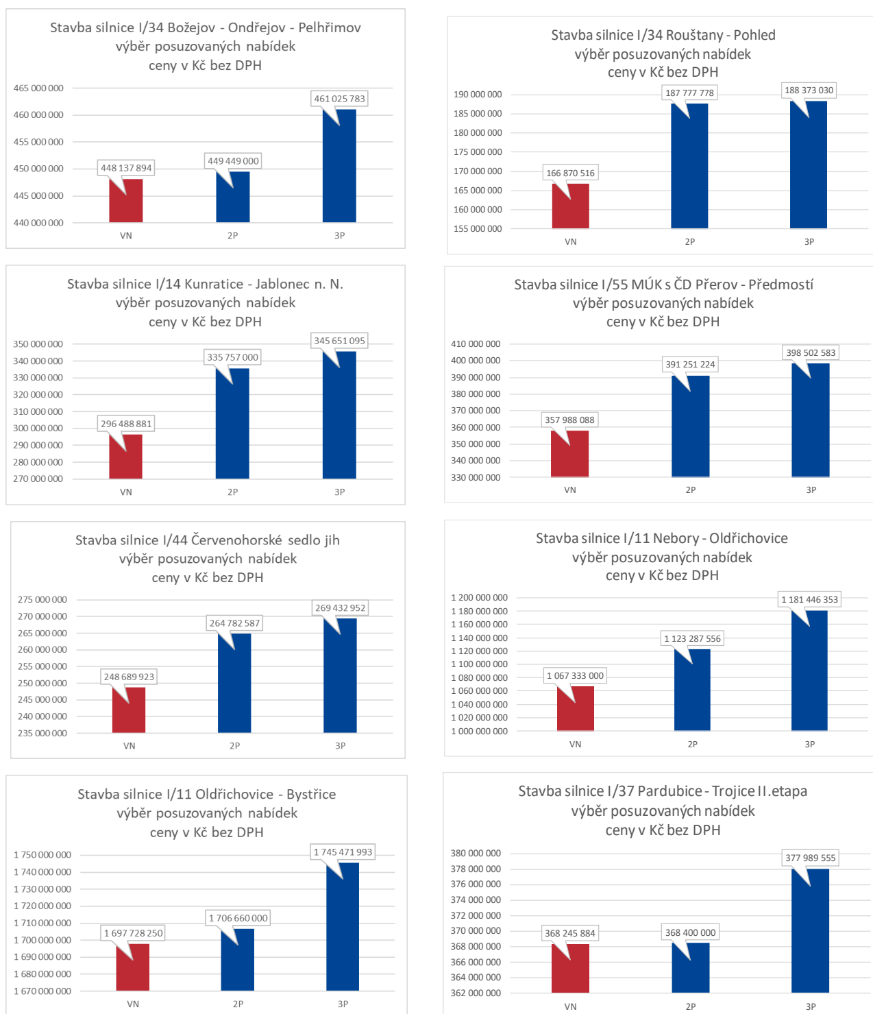
Graf č. 3-11: Rozptyl nabídkových cen z veřejných soutěží na stavby silnic I. třídy
